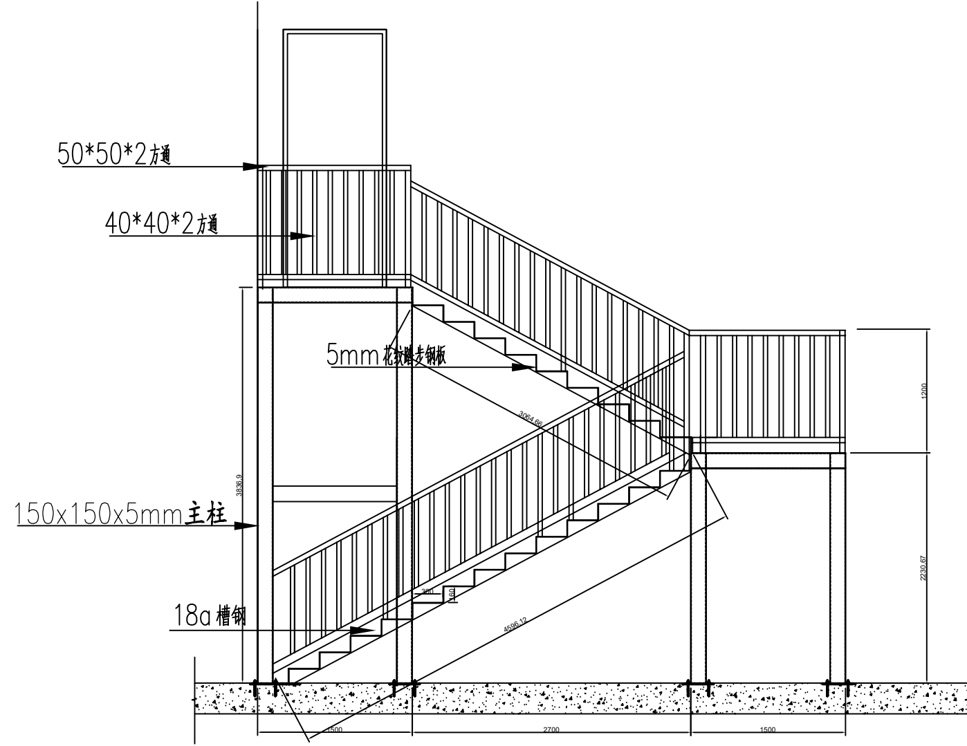
固定钢结构斜梯剖面图
