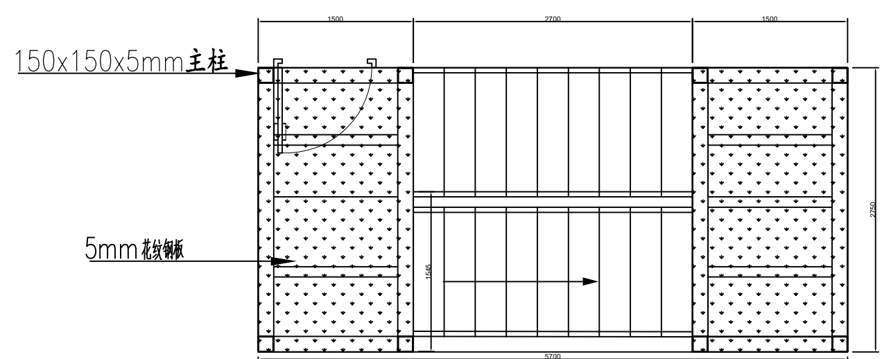
固定钢结构斜梯平面图
